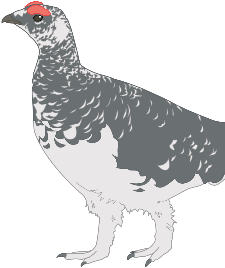
Das Alpenschneehuhn ist besonders stark vom Klimawandel betroffen. 38
