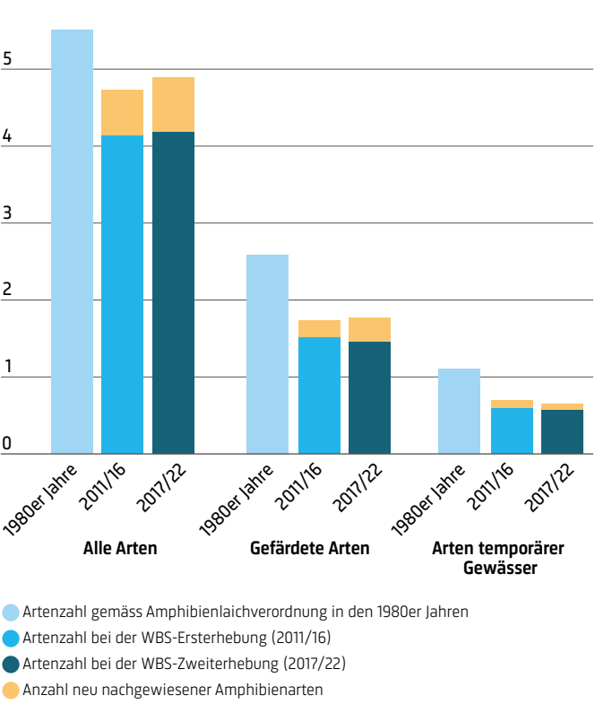
6 Mittlere Artenzahl pro Amphibienlaichgebiet
