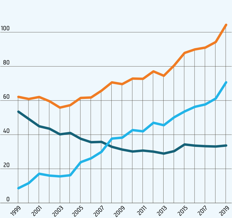
120 Anzahl besiedelter Weiher
